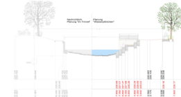
Schnitt B-B
